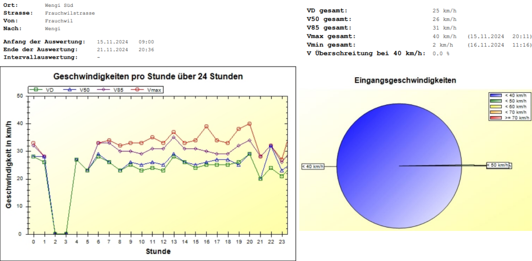
Abbildung 27: V 85, Vmax und V Überschreitung bei dem Tempolimit 40, Frauchwilstrasse, Punkt e. Quelle: Messungen der Gemeinde Wengi zwischen 15.11 und 21.11.2024 (von Frauchwil nach Wengi).
