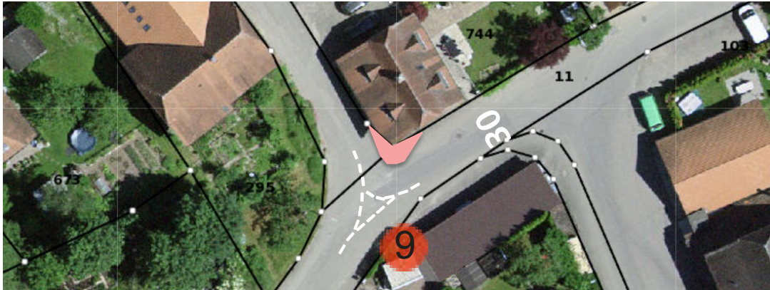
Illustration der Massnahmen: Tempo-30-Zone, Tulpe und Einengung.
