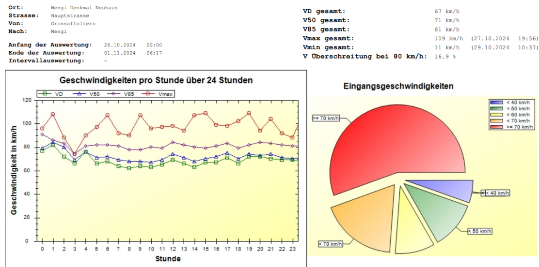
Abbildung 24: V 85, Vmax und V Überschreitung bei dem Tempolimit 80, Hauptstrasse (Neuhaus), Punkt b. Quelle: Messungen der Gemeinde Wengi zwischen 26.10. und 01.11.2024 (von Grossaffoltern nach Wengi).
