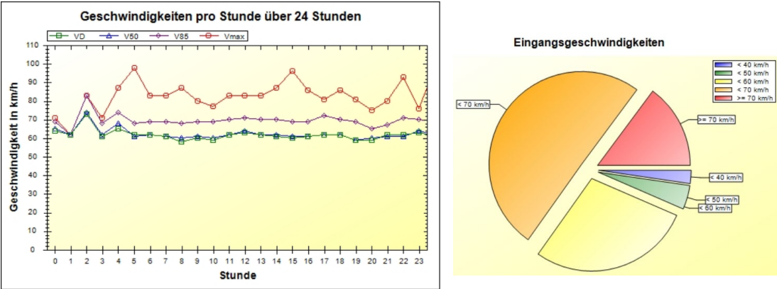
Abbildung 26: V 85, Vmax und V Überschreitung bei dem Tempolimit 60, Hauptstrasse-Reuentalstrasse, Punkt d. Quelle: Messungen der Gemeinde Wengi zwischen 02.10 und 04.10.2024 (von Messen nach Wengi).
