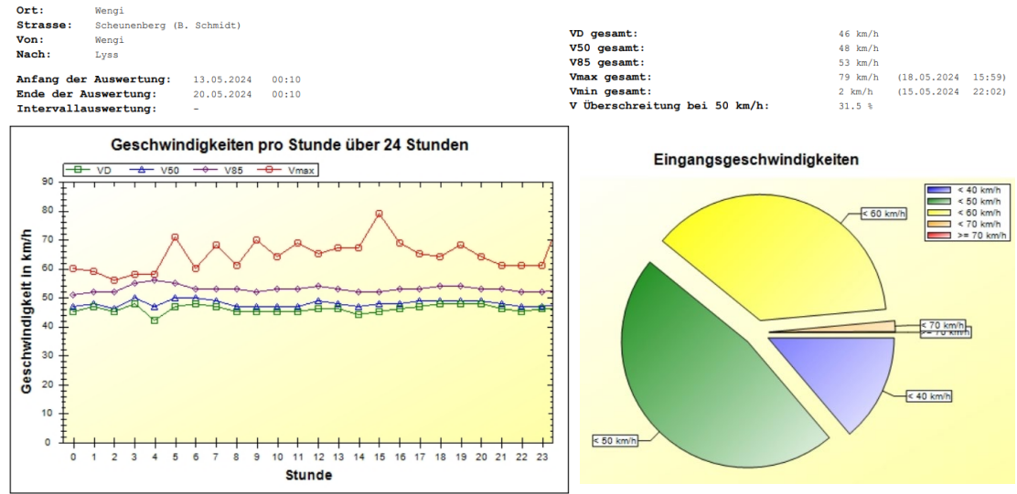
Abbildung 22: Vmax und V Überschreitung bei dem Tempolimit 50, Punkt j. Quelle: Messungen der Gemeinde Wengi zwischen 13.05 und 20.05.2024.
