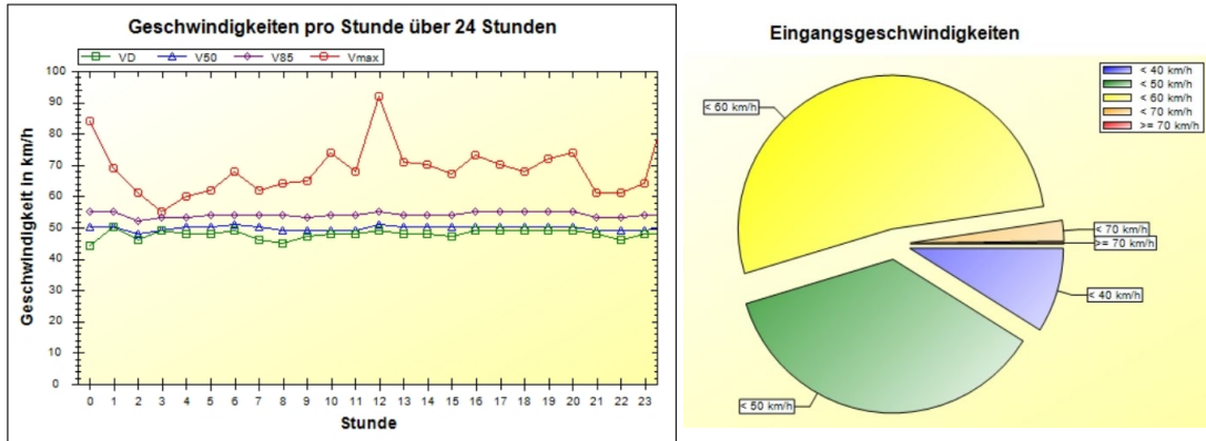
Abbildung 23: Vmax und V Überschreitung bei dem Tempolimit 50, Punkt h, Hauptstrasse. Quelle: Messungen der Gemeinde Wengi zwischen 21.04 und 24.04.2024.
