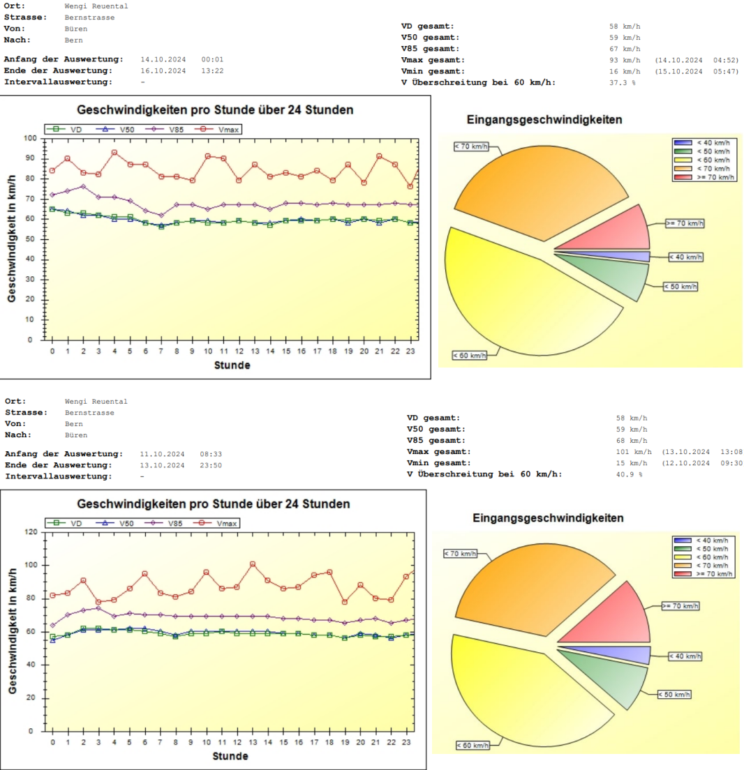
Abbildung 25: V 85, Vmax und V Überschreitung bei dem Tempolimit 60, Bernstrasse, Punkt c. Quelle: Messungen der Gemeinde Wengi zwischen 11.10 und 13.10.2024 (von Bern nach Büren) und zwischen 14.10.-16.10.2024 (von Büren nach Bern).
