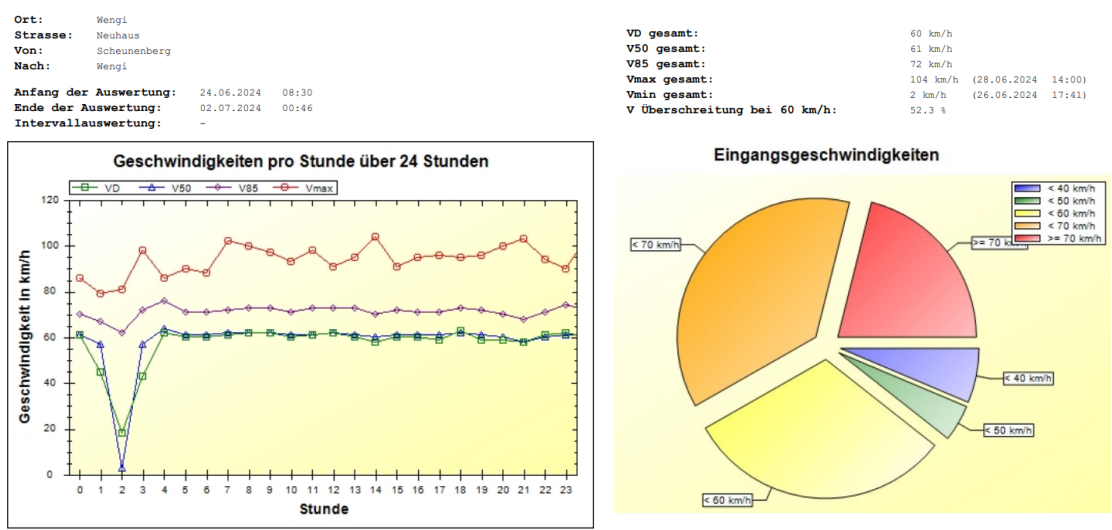
Abbildung 21: Geschwindigkeitsüberschreitungen an Punkt a (südlich der Strasse Scheunenberg) mit Vmax und V Überschreitung bei dem Tempolimit 60. Quelle: Messungen der Gemeinde Wengi zwischen 24.06 und 02.07.2024.
