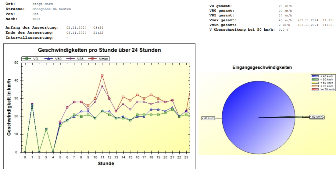
Abbildung 28: V 85, Vmax und V Überschreitung bei dem Tempolimit 50, Moosgasse, Punkt f. Quelle: Messungen der Gemeinde Wengi zwischen 02.11. und 05.11.2024 (von Ost nach West).
